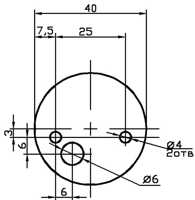
Габаритные и установочные размеры устройства доступа УД-3Т
