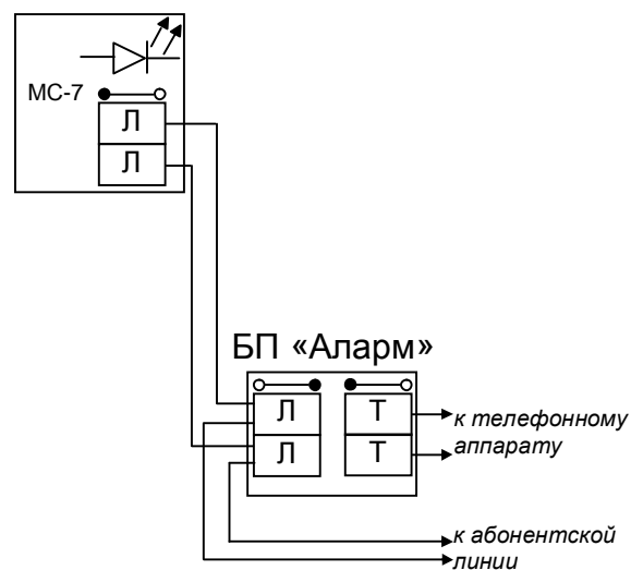
б) схема подключения МД-7
