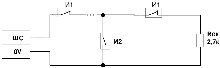
а) при контроле состояния ШС без выделения сработки ПИ
