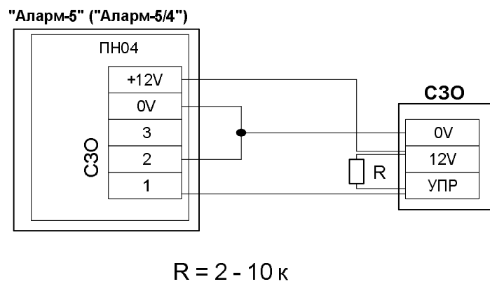
Рисунок 5 - Схемы подключения к реле С30 приборов внешнего С30 со встроенной АКБ и управляющей цепью
