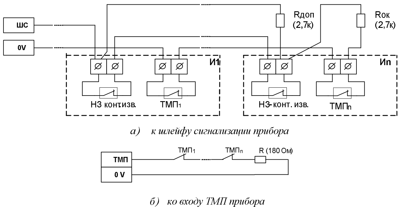
Рисунок 6 - Схема подключения нормально - замкнутых тампер - контактов внешних устройств
