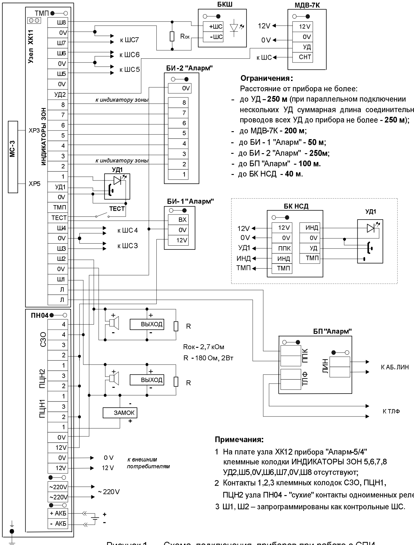
Рисунок 1 - Схема подключения приборов при работе с СПИ
