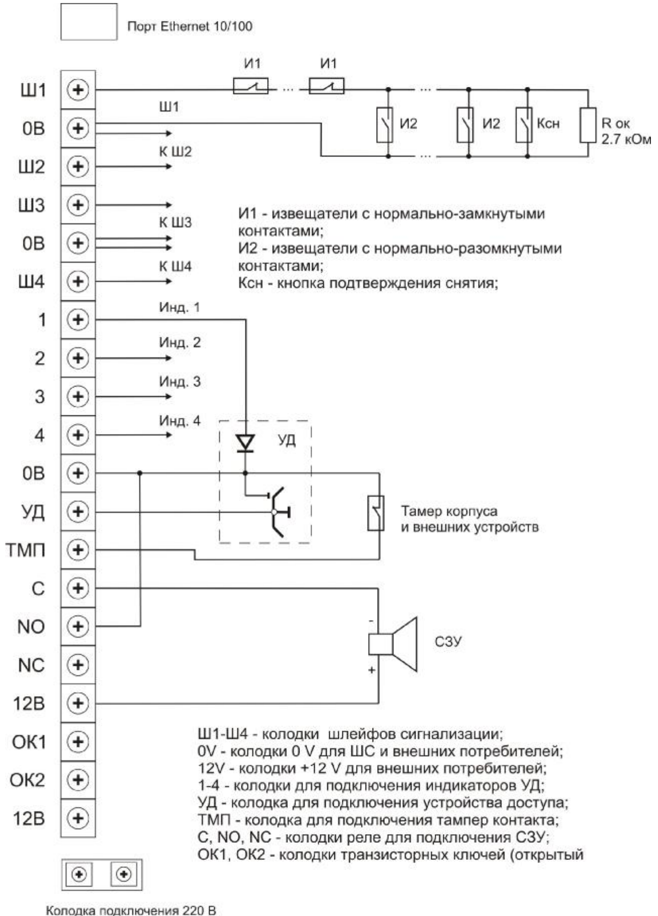
Рисунок 6. Схема подключения прибора
