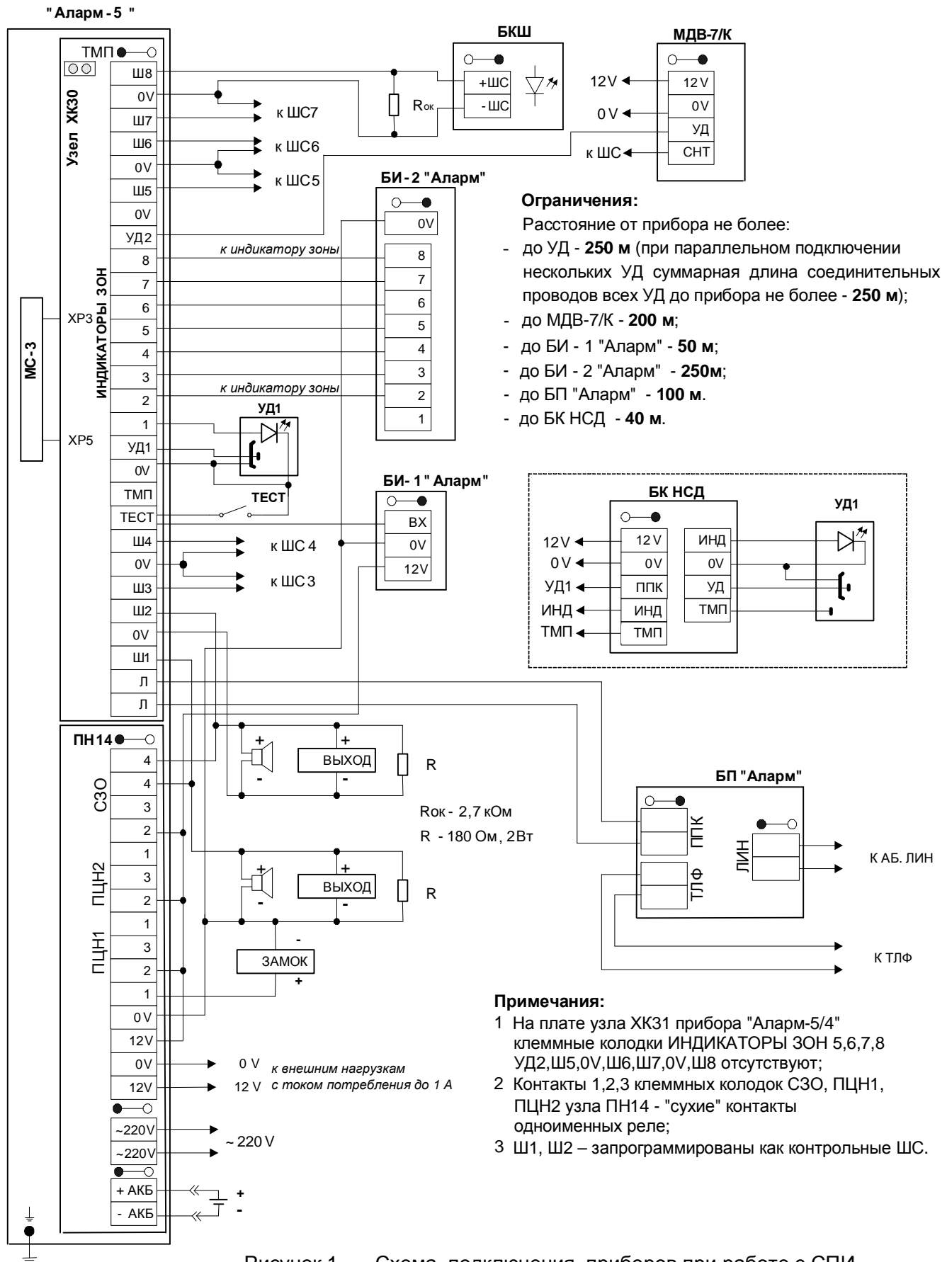
Рисунок 1 - Схема подключения приборов при работе с СПИ
