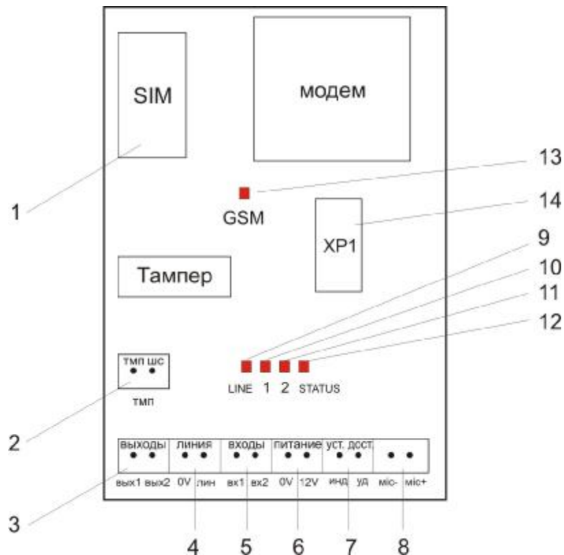
Рисунок 1 – Схема расположения элементов на узле функциональном модуля
