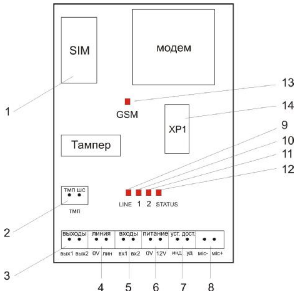
Рисунок 1 – Схема расположения элементов на узле функциональном модуле
