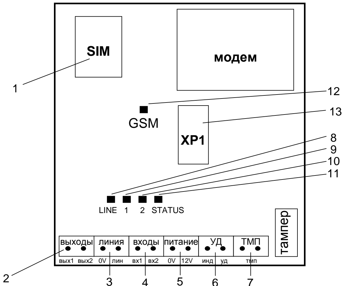
Рисунок 1 – Схема расположения элементов на узле функциональном модуля
