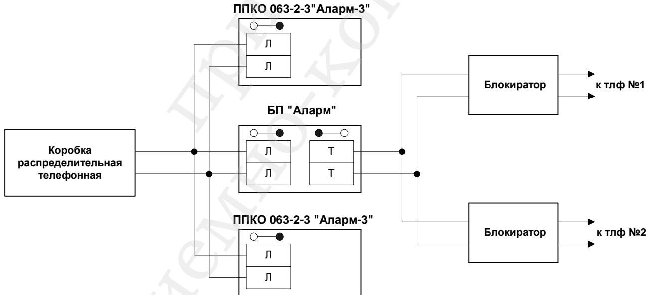
б) с использованием одного БП "Аларм"
