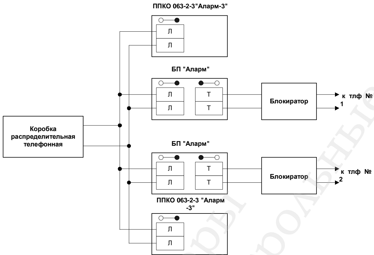
а) с использованием двух БП "Аларм"
