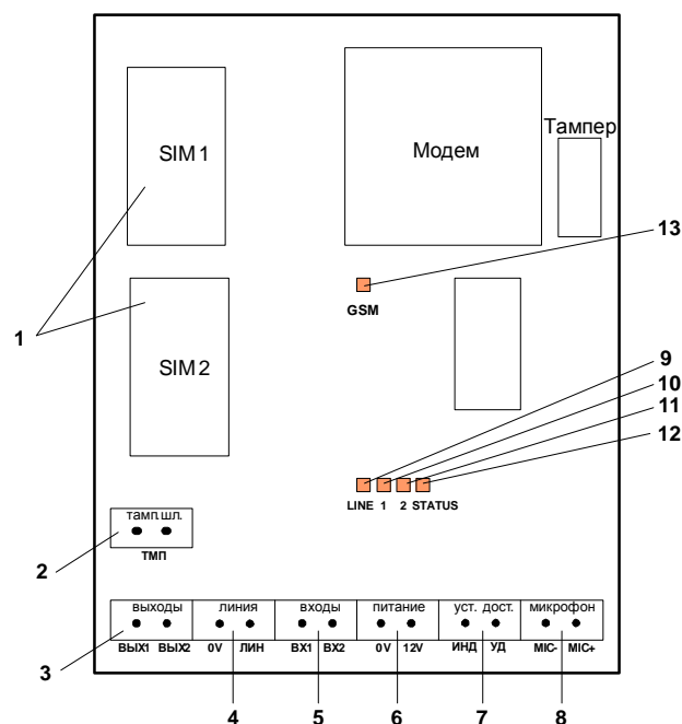
Рисунок 1 – Схема расположения элементов на узле функциональном модуля а) соединители «SIM1», «SIM2» (обозначение 1) – для установки SIM-карт;
