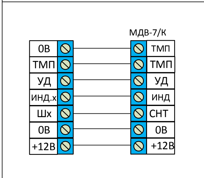
Рис.7 Схема подключения МДВ-7/К*
