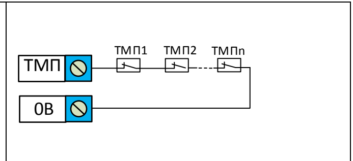
Рис.4 Схема подключения тамперов
