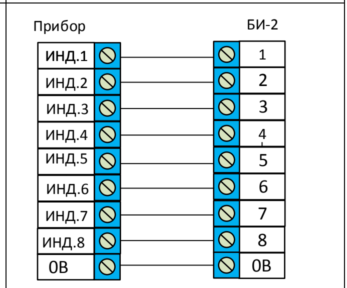
Рис.8 Схема подключения БИ-2
