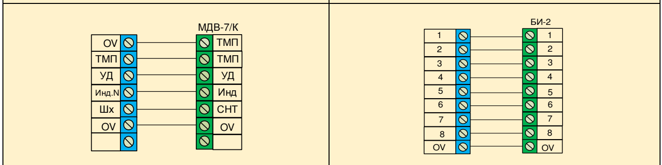
Рис.7 Схема подключения МДВ-7/К*
