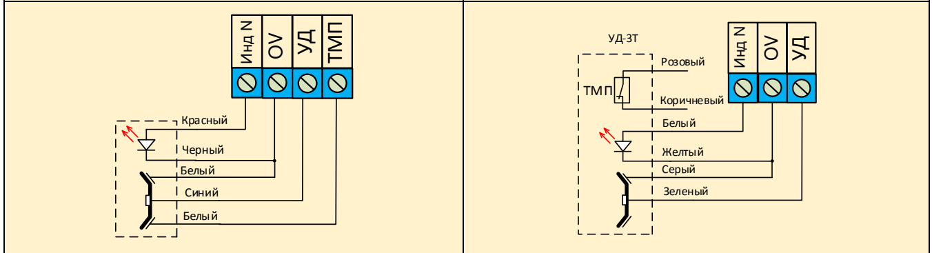
Рис.5 Схема подключения УД-1Т*
