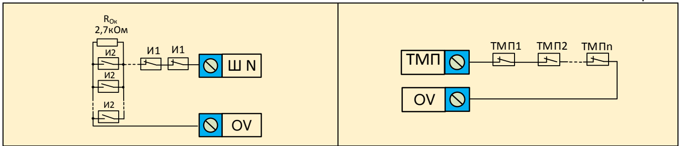
Рис.4 Схема подключения тамперов
