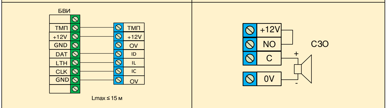
Рис.9 Схема подключения БВИ
