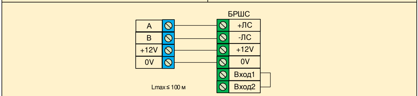
Рис.11 Схема подключения БРШС
