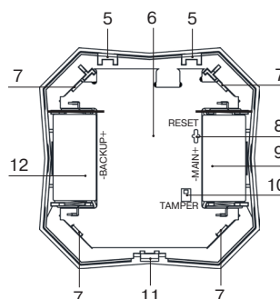
Рисунок 2 – Конструкция «Трубоч-РК»
