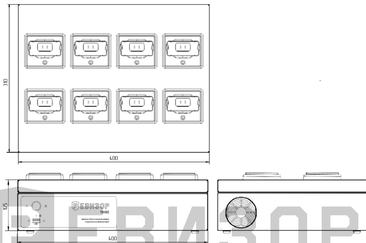
Рисунок 1 – Габаритные размеры терминала Т8HDD/Т12HDD
