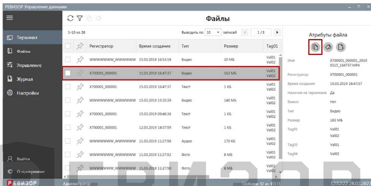
Рисунок 41 – Вызов команды копирования одного «Файла»
