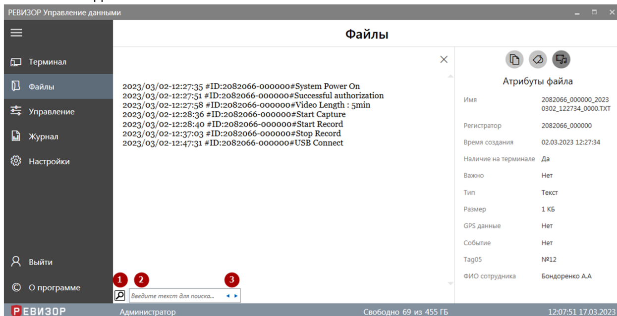
Рисунок 46 – Поиск по содержимому текстового файла
