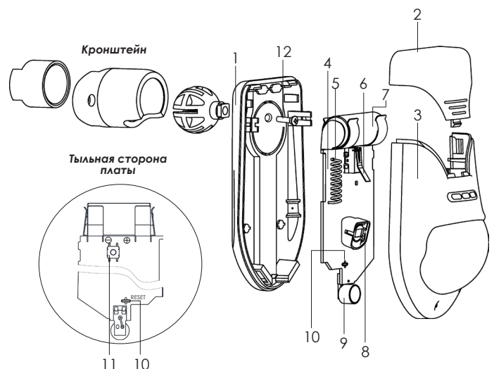
Рисунок 3 – Конструкция датчика
