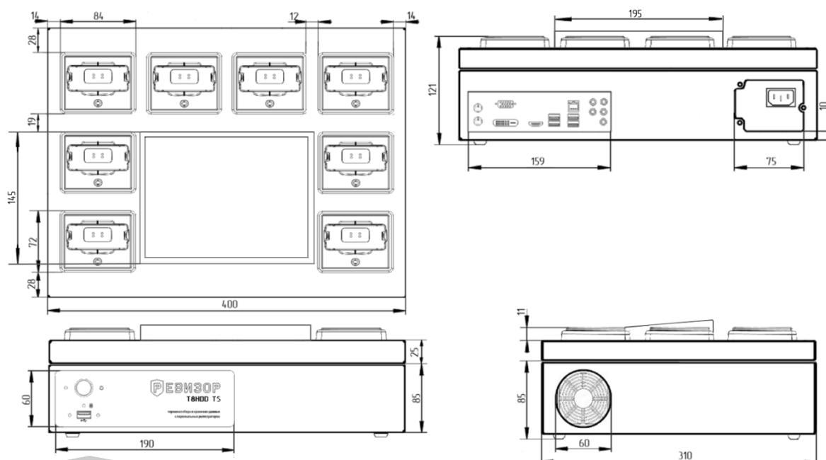
Рисунок 1 – Габаритные размеры терминала T8HDD TS
