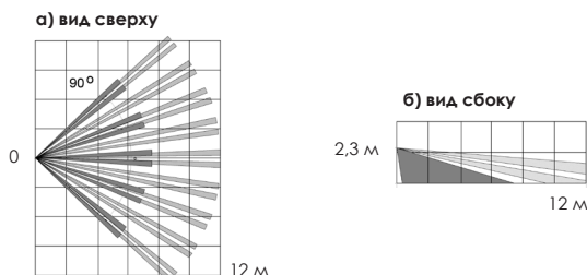
Рисунок 2 – Диаграмма зоны обнаружения
