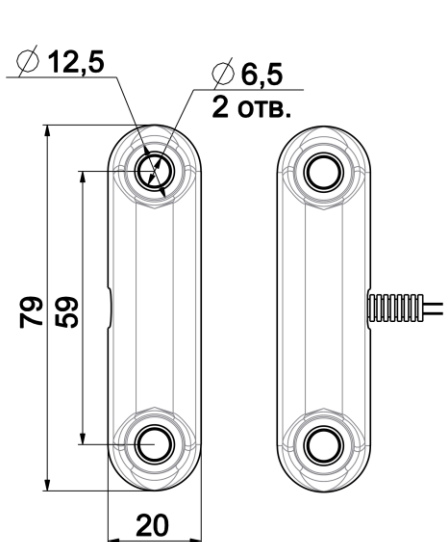
Рис. 1. Габаритные и установочные размеры: исполнительный блок – 79x20x18. задающий блок – 79x20x18.
