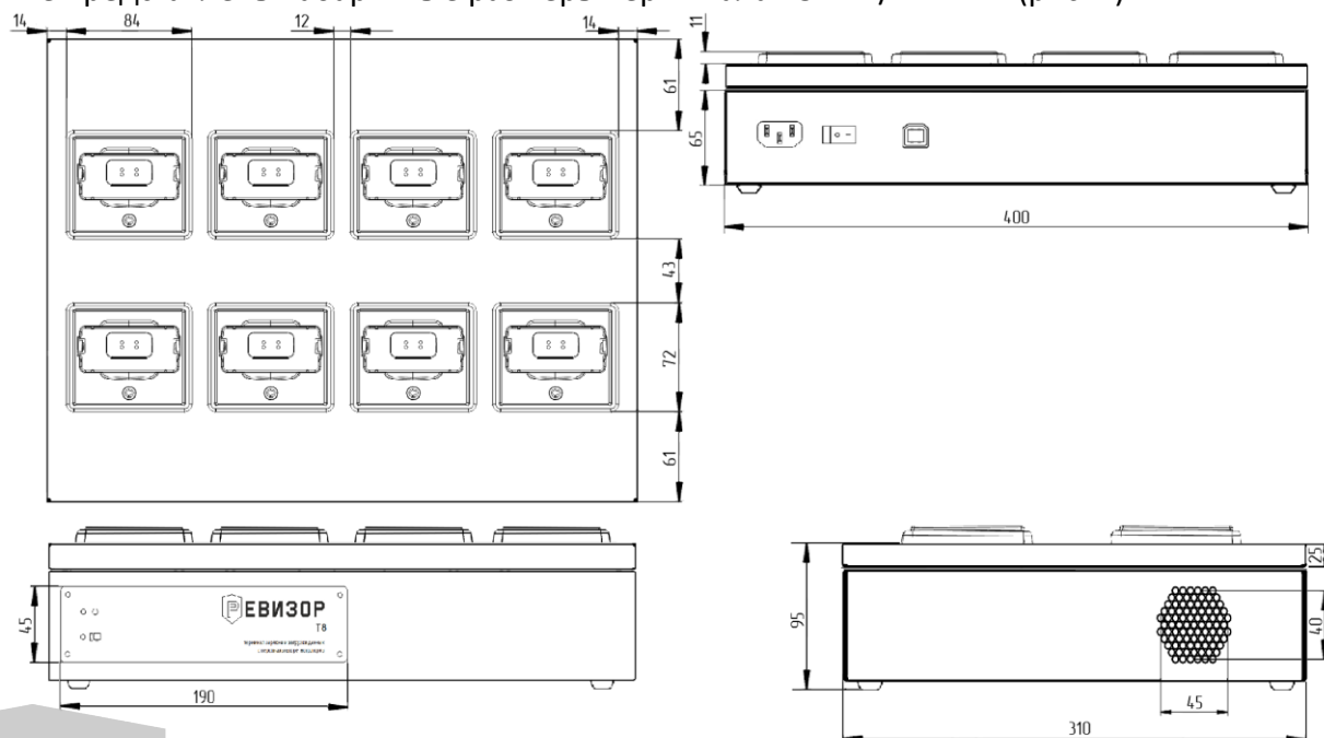
Рисунок 1 – Габаритные размеры терминала Т8/Т12
