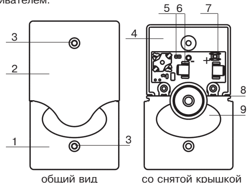
Рисунок 2 – Корпус оповещателя
