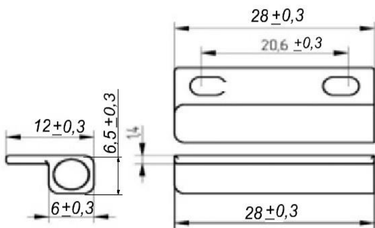
Рис.1. Габаритные и установочные размеры
