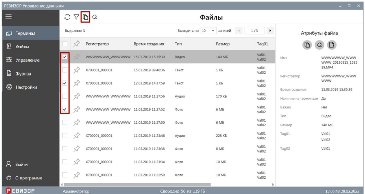
Рисунок 43 – Вызов команды массового копирования «Файлов»
