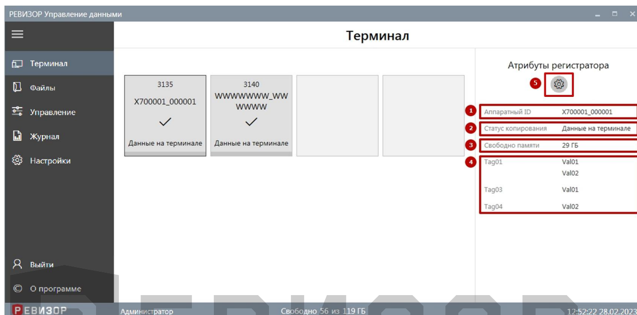
Рисунок 19 – Просмотр атрибутов регистратора (раздел «Терминал»)
