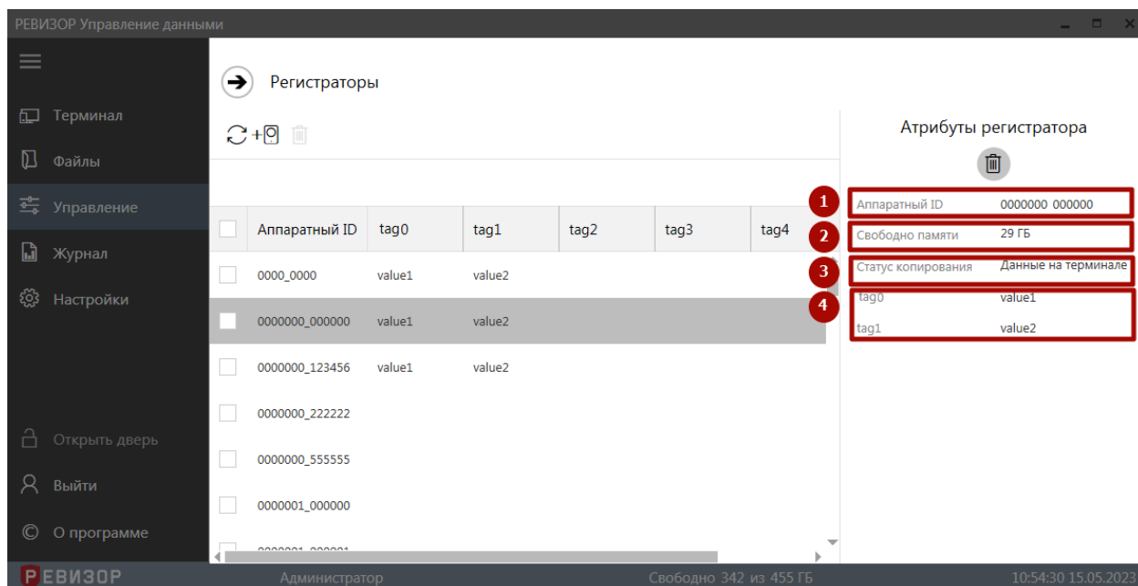
Рисунок 20 – Просмотр атрибутов регистратора (раздел «Управление»)
