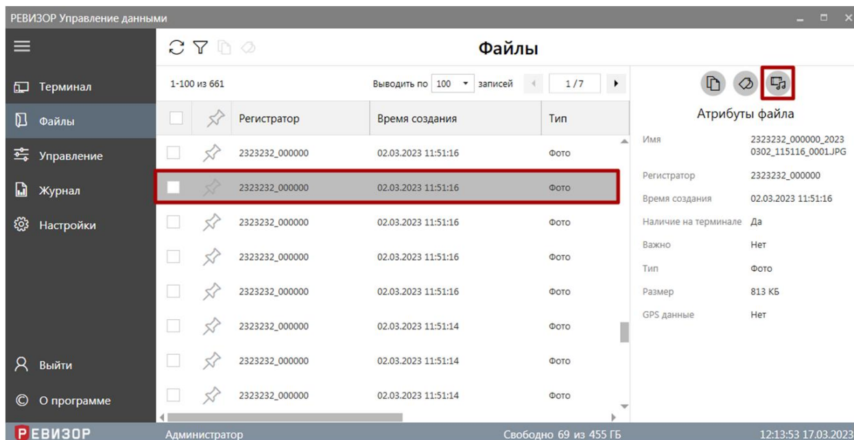
Рисунок 50 – Вызов просмотра содержимого «Файла» с типом Фото
