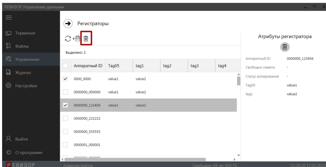
Рисунок 89 – Массовое удаление «Регистраторов»
