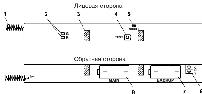
Рисунок 1 – Корпус оповещателя
